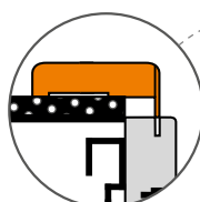
SCHEMAT UMIEJSCOWIENIA ELEMENTÓW POSZERZEŃ OŚCIEŻNICY DO SYSTEMU PRZESUWNEGO CHOWANEGO W ŚCIANĘ
