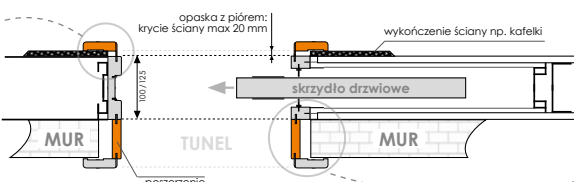
SCHEMAT UMIEJSCOWIENIA ELEMENTÓW POSZERZEŃ OŚCIEŻNICY DO SYSTEMU PRZESUWNEGO CHOWANEGO W ŚCIANĘ
